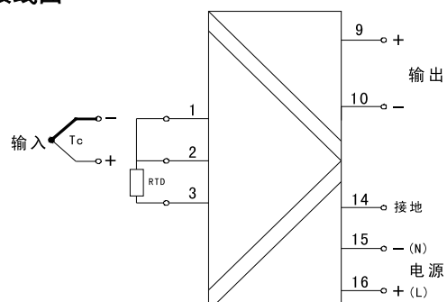
热电偶/热电阻输入, 单输出
