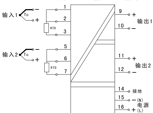
双路热电偶/热电阻输入, 双输出
